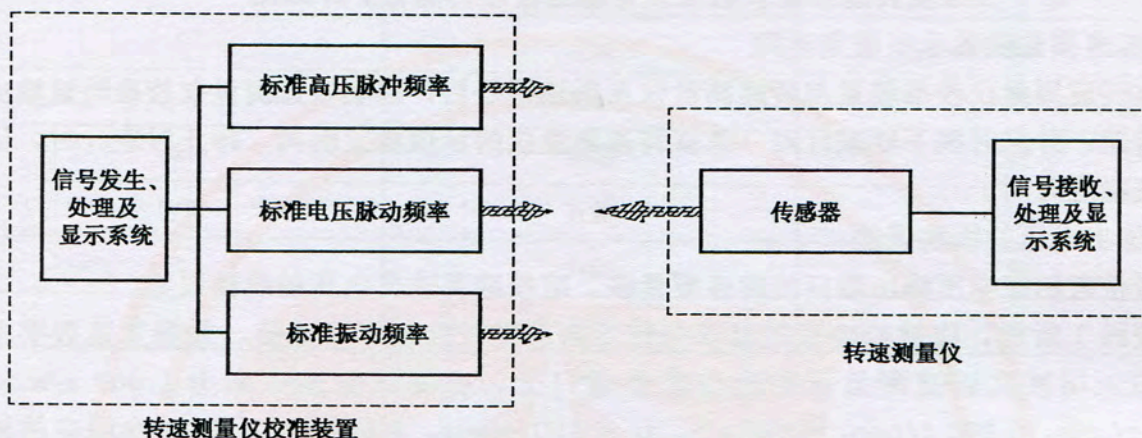
图 1 转速测量仪校准方法示意图
